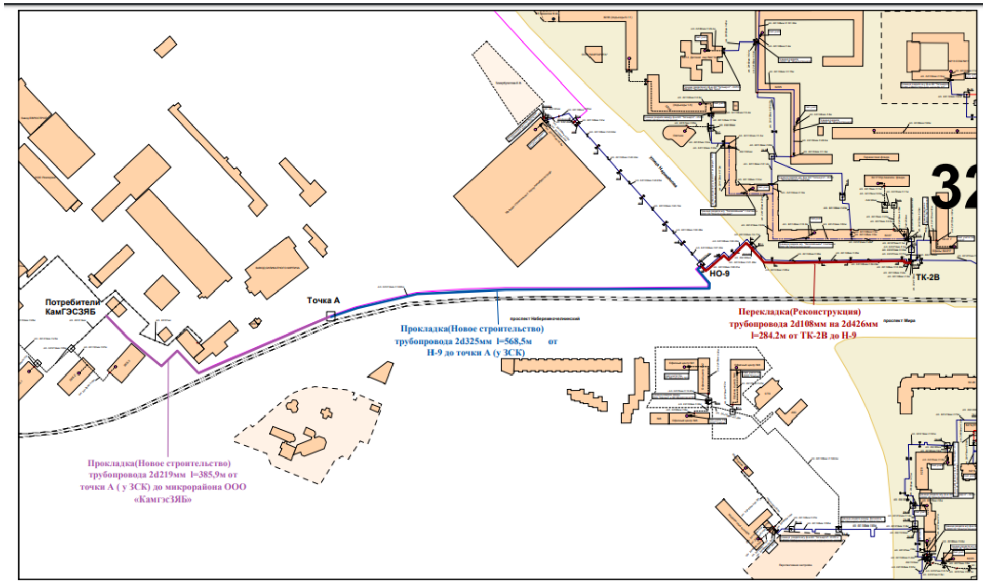
Рис. 8.1 Схема подключения потребителей ООО «Камгэс – ЗЯБ» к тепловым сетям «НЧТС».
